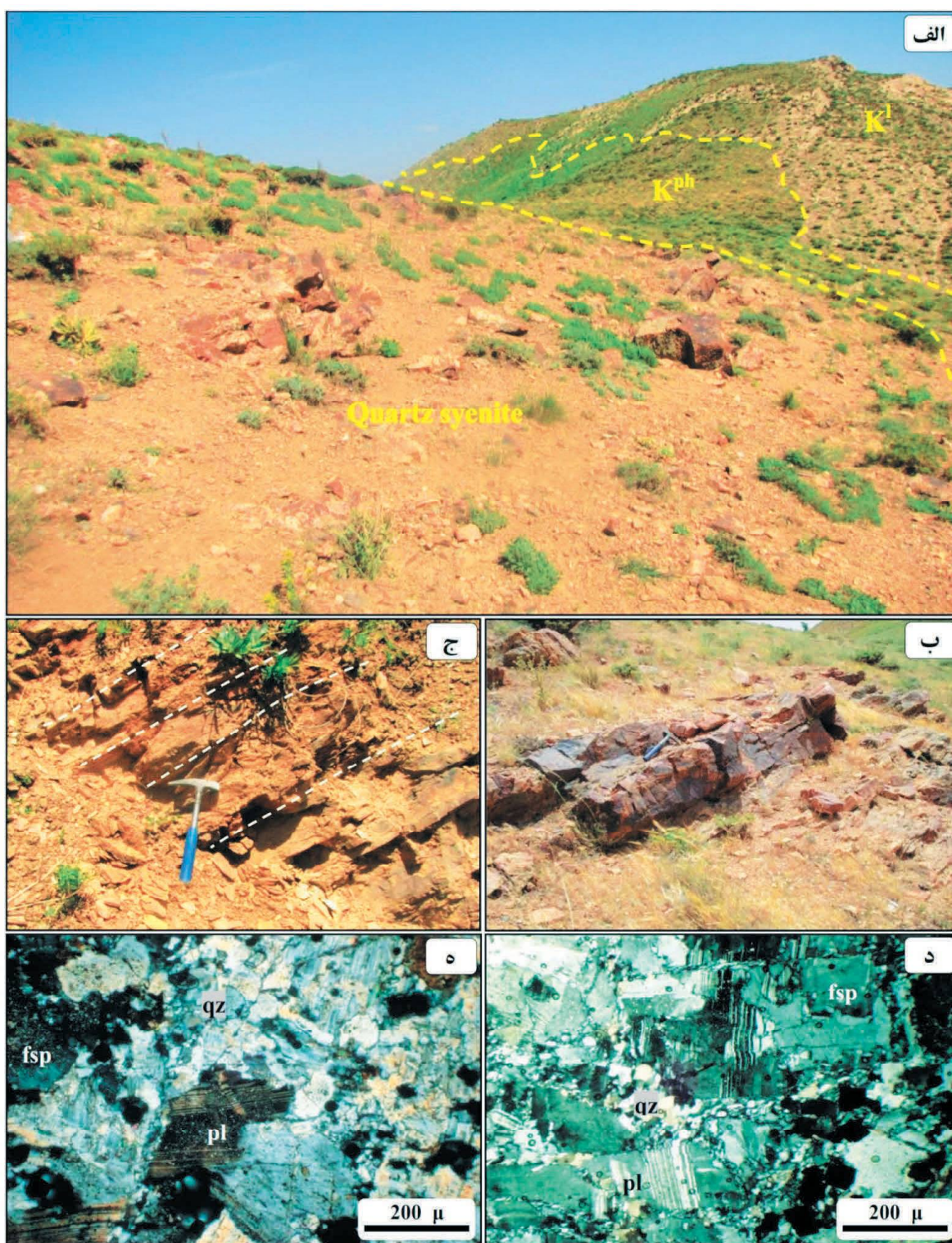
شکل ۳. موقعیت زمین‌شناسی و پتروگرافی توده گرانیتوئیدی میزبان کانی‌سازی طلا در محدوده غرب کسنزان، الف) توده کوارتز سینیتی در داخل واحد فیلیتی ( K^{ph} ) که دربردارنده یک میان‌لایه آهکی ( K^1 ) است، نفوذ کرده است، ب، ج) نمای نزدیک‌تر از برونزدهای کوارتز سینیتی، که به شدت میلونیتی و دگرسان بوده و با برگوارگی میلونیتی همراه شده‌اند، د، ه) تصاویر میکروسکوپی از توده کوارتز سینیتی، که فابریک‌های دگرشکلی از جمله تبلور مجدد دینامیکی در بلورهای کوارتز و جایجایی ماکلی و نیز خمیدگی در پلاژیوکلازها را نشان می‌دهد. تصاویر میکروسکوپی در نور عبوری با نیکول‌های متقاطع (XPL) برداشت شدند. نشانه‌های اختصاری کانی‌ها از (Whitney and Evans 2010) اقتباس شده است. fsp: فلدسپار، pl: پلاژیوکلاز و qz: کوارتز
