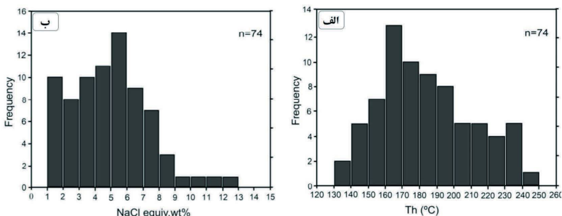
شکل ۸. الف) نمودار دماهای همگن شدن به فراوانی میان‌بارهای سیال، ب) نمودار درجه شوری به فراوانی میان‌بارهای سیال در کانی‌های کوارتزی موجود در کانسنگ طلا در محدوده غرب کسنزان
