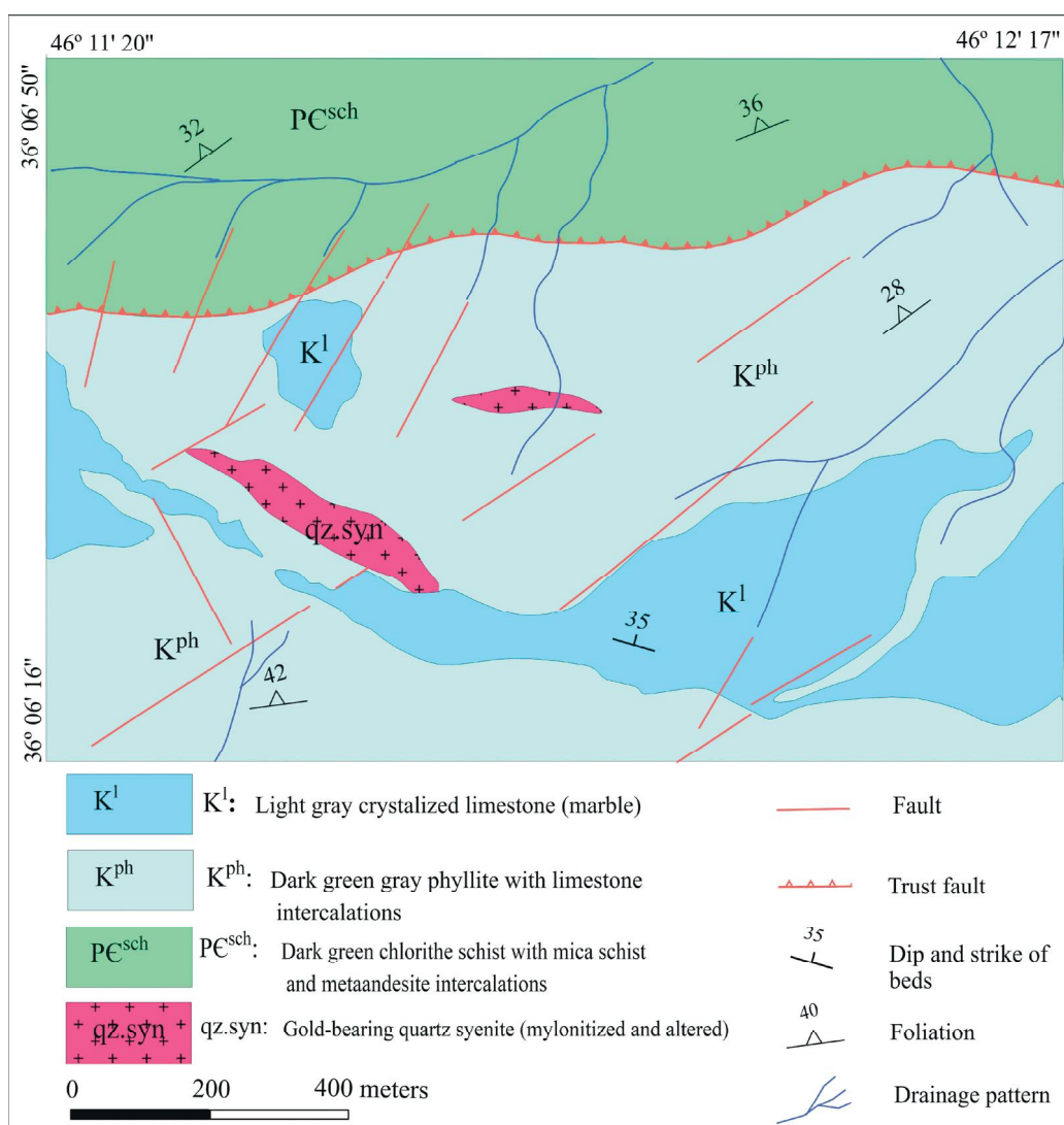
شکل ۲. نقشه زمین‌شناسی غرب گستره کسنزان. توده گرانیتوئیدی اصلی، با راستای شمال غرب، جنوب شرق در واحد K ph تزریق شده است (تاج‌الدین، ۱۳۹۰)
